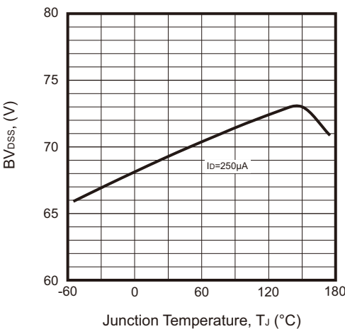
Fig.10 - BV_{DSS} vs T_J
